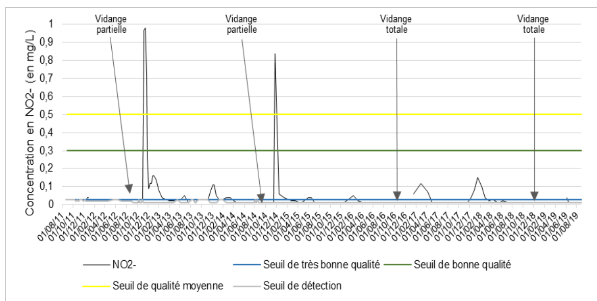
Figure 27 : Evolution de la concentration en nitrites (en mg/L de \text{NO}_2^- ) d'août 2011 à août 2019
