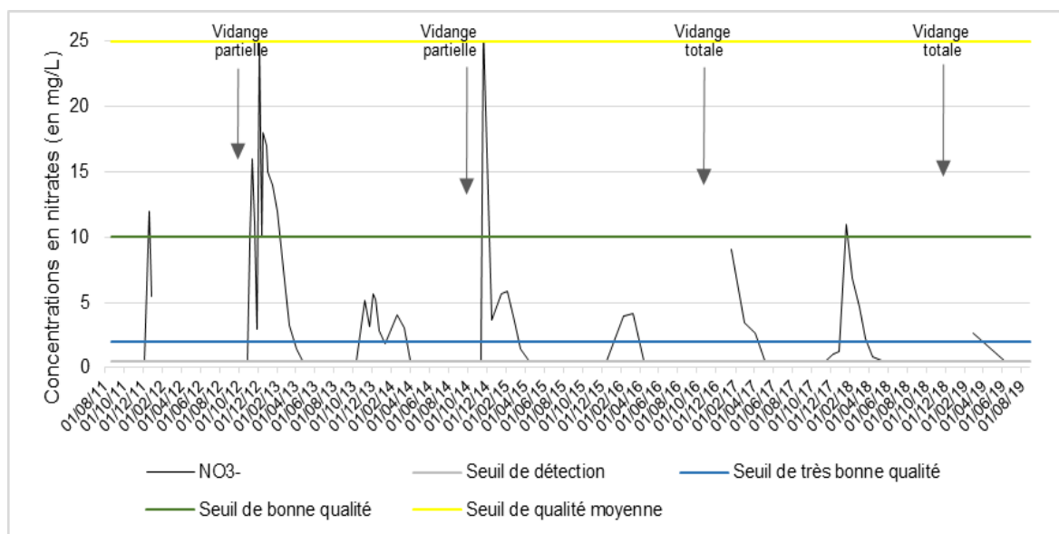
Figure 29 : Evolution de la concentration en nitrates (en mg/L de \text{NO}_3^- ) d'août 2011 à août 2019
