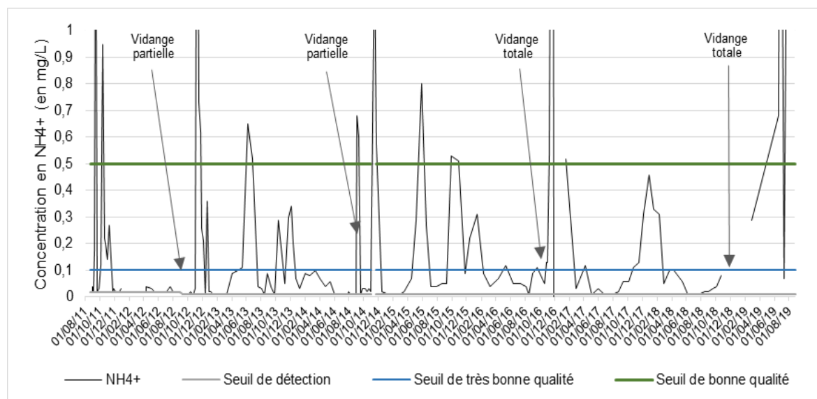
Figure 26 : Evolution de la concentration en ammonium (en mg/L de \text{NH}_4^+ ) d'août 2011 à août 2019
