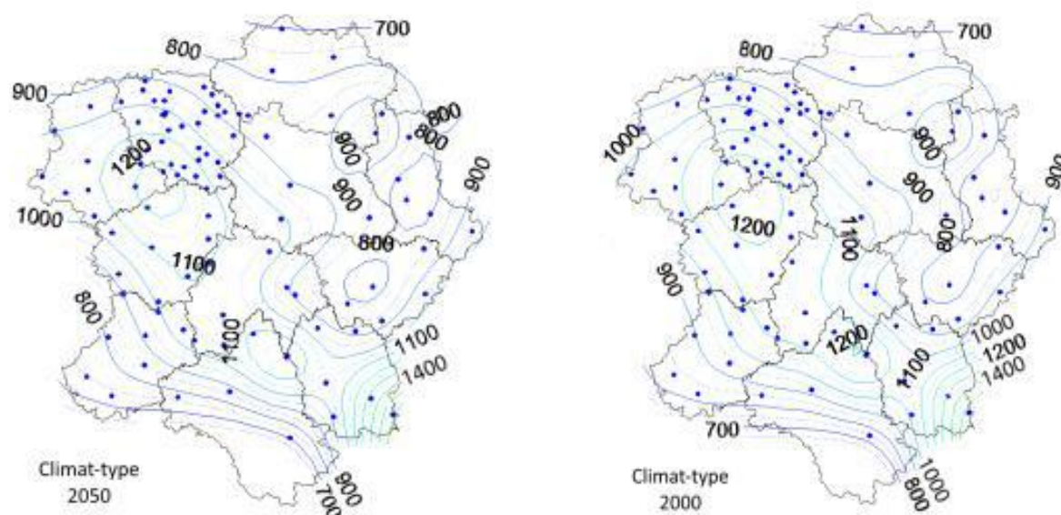
Figure 7 : Cumul de précipitations (carte des isohyètes en mm) sur le Massif central de 2000 à 2050 (cartes réalisées dans le cadre du projet AP3C et fournies gracieusement)
