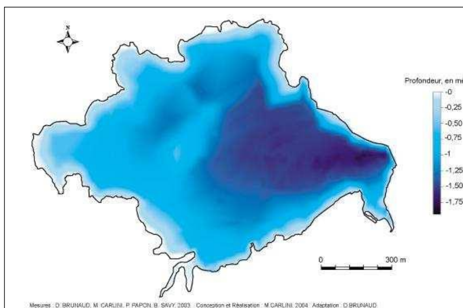
Figure 21 : Bathymétrie de l'étang des Landes (Source : D. BRUNAUD, 2004)
